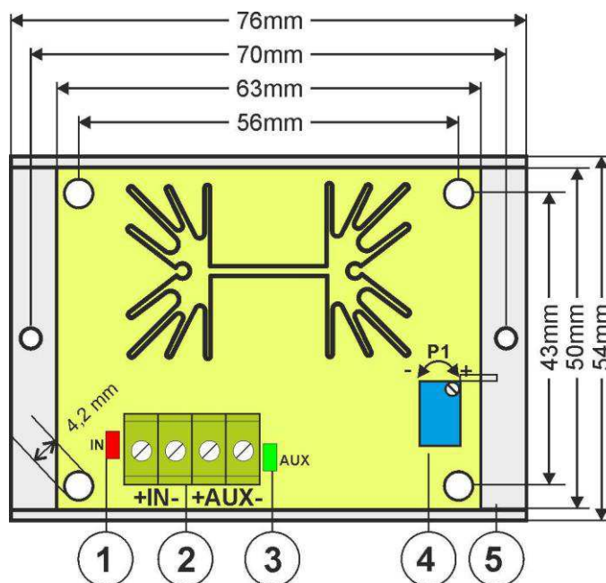
Rys.3. Widok reduktora napięcia RN250.
