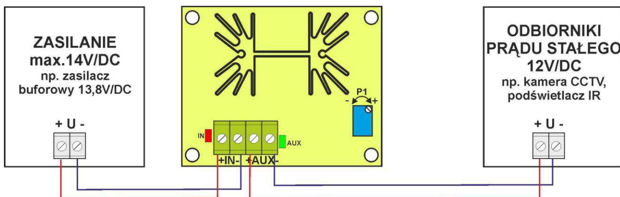
Rys.2. Typowa aplikacja zastosowania reduktora napięcia RN250.
